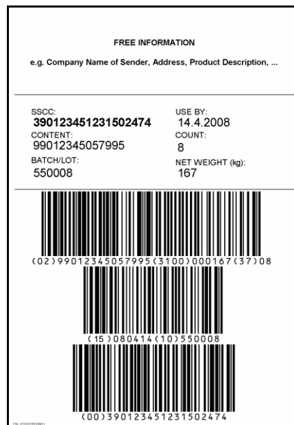
Abbildung: Transportetikett für sortenreine Palette mit gewichtsvariablem Artikel
